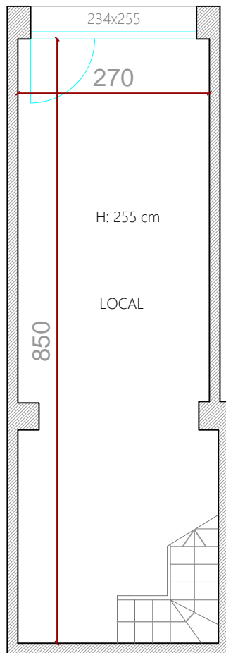
PLANTA BAJA
